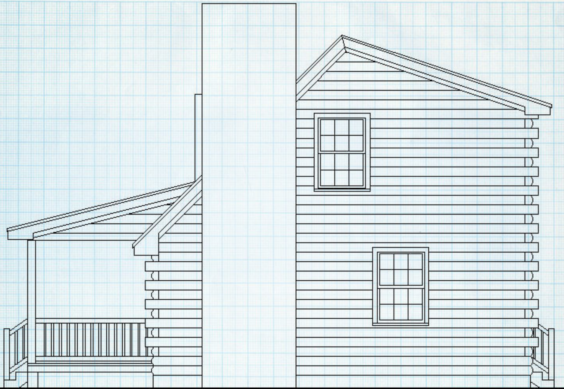
RIGHT ELEVATION
