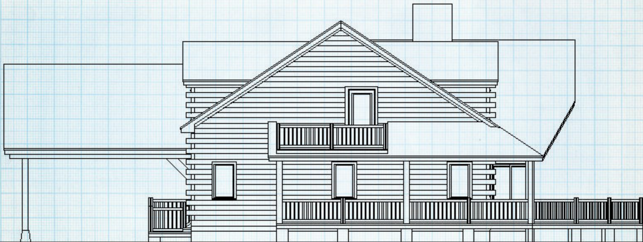
RIGHT ELEVATION
