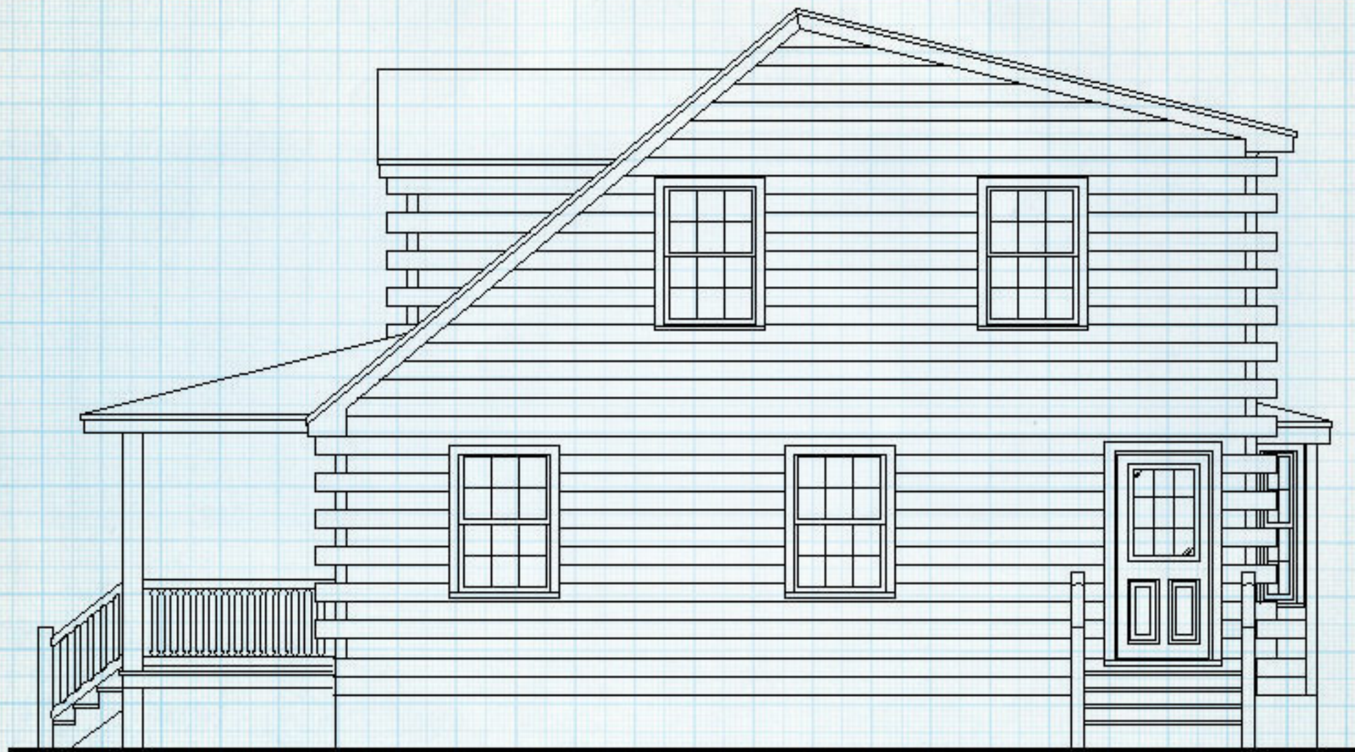
RIGHT ELEVATION
